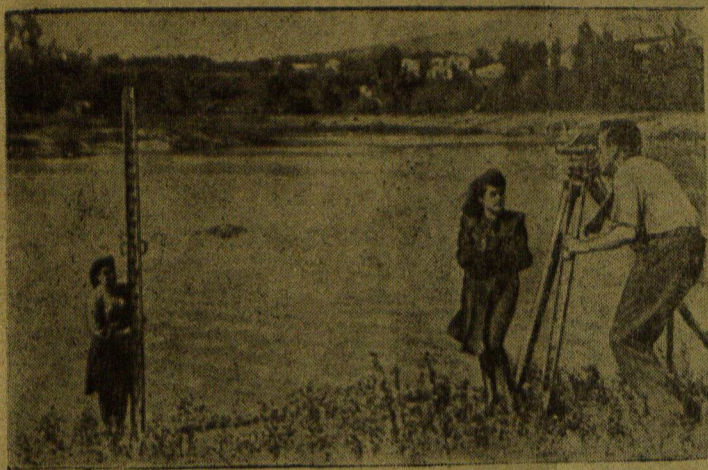
Строительство водного бассейна в парке культуры и отдыха. На снимке: инженер «Севкавводпроекта» Р. Саркисян со своими помощниками за нивелировочной работой. Фото В. Зильберга.
